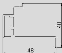
profiel
